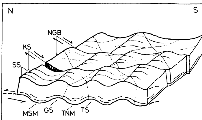
Abb. 9: NGB – Nassereither Grenzblatt, KS – Kratzerstörung, MSM – Mutterkopfgosau-Sinnesbrunnmulde, GS – Gurgltalsattel, TNM – Tschirgant-nordmulde, TS – Tschirgantsattel
